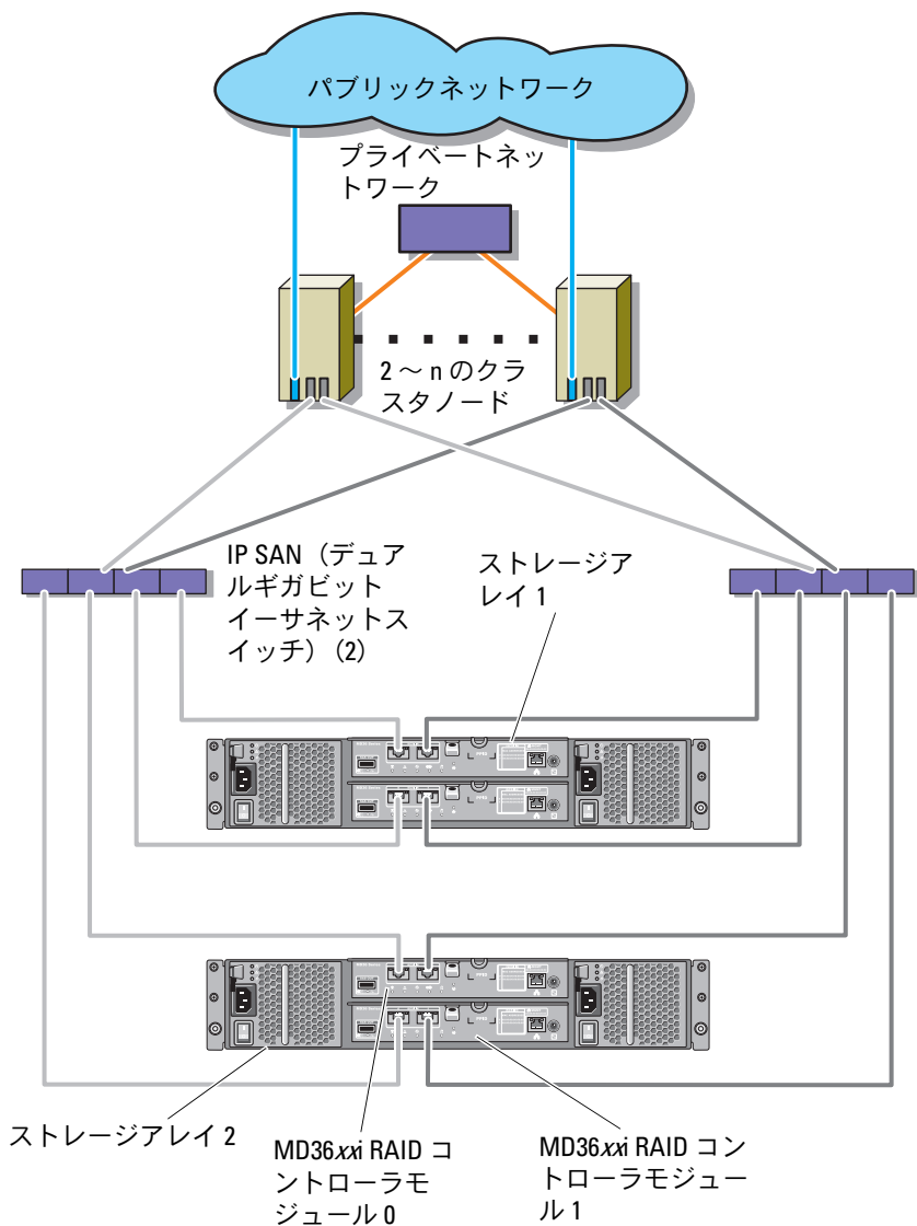
図 2-5. 複数のストレージレイを使用したネットワーク接続のクラスタ構成
