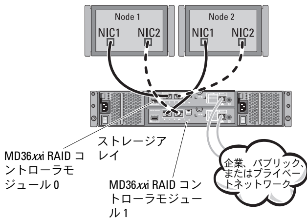
図 1-1. 直接接続のクラスタ構成
