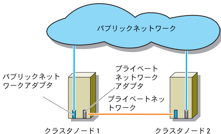
図 2-2. ネットワークのケーブル接続の例
