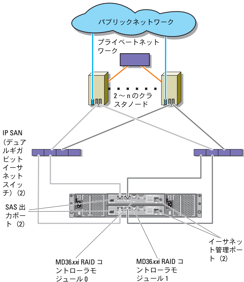
図 2-4. ネットワーク接続のクラスタ構成
