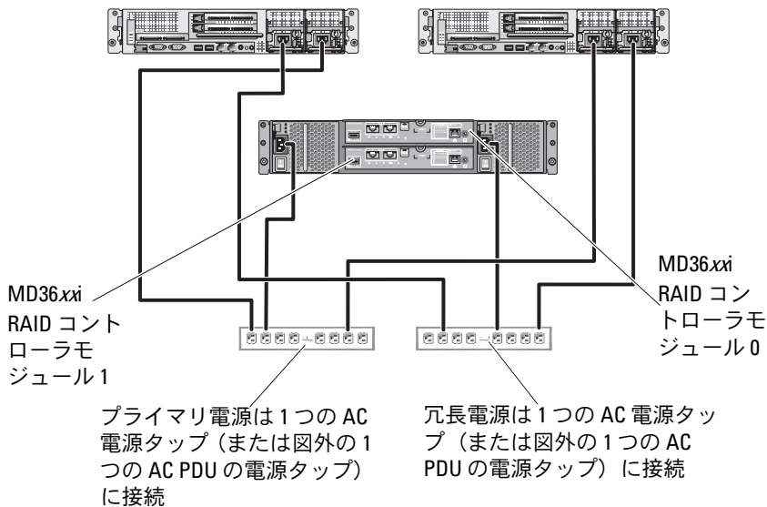
図 2-1. 電源ケーブルの接続例
