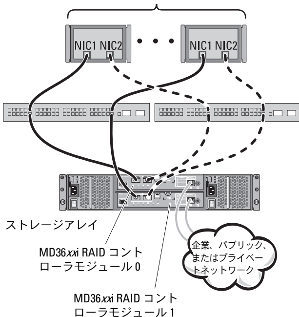
図 1-2. ネットワーク接続の冗長クラスタ構成
